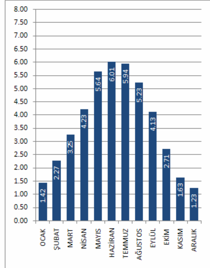
SİNOP İLİ GLOBAL RADYASYON DEĞERLERİ (KWh/m 2 -gün)
