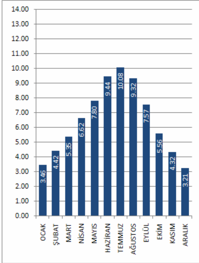
SİNOP İLİ GÜNEŞLENME SÜRESİ DEĞERLERİ (Saat)
