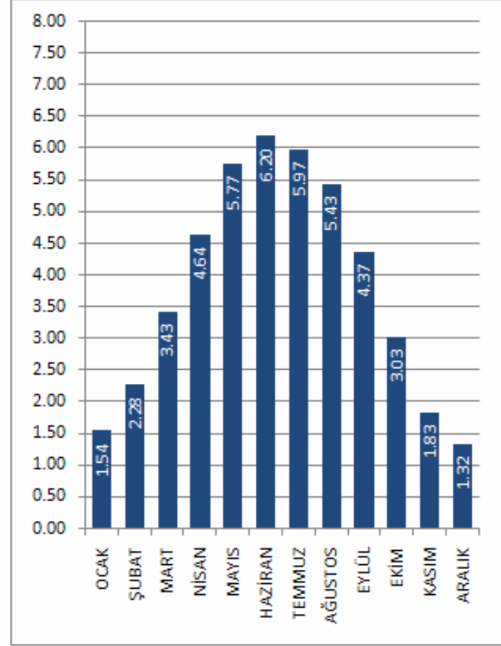
BURSA İLİ GLOBAL RADYASYON DEĞERLERİ (KWh/m 2 -gün)
